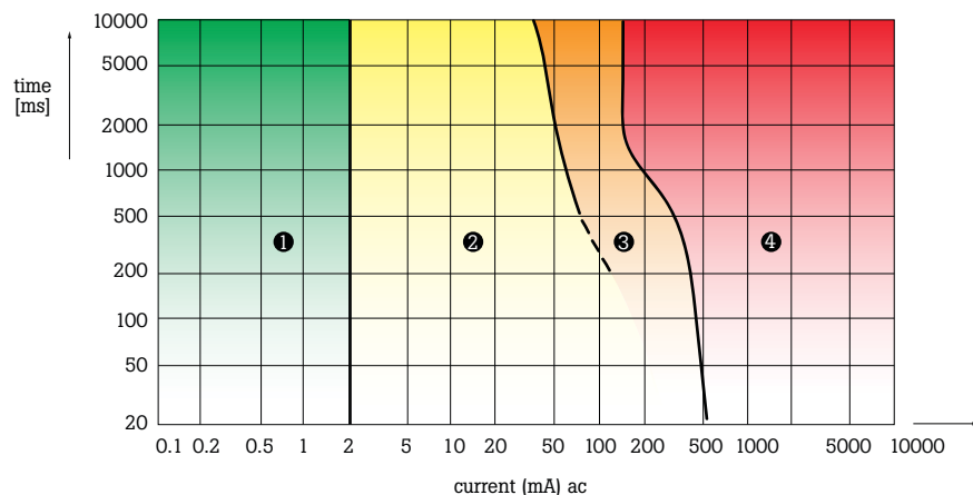
Abbildung 2: Auswirkung von Wechselstrom (bei Effektivwerten von 50 bis 60 Hz)
